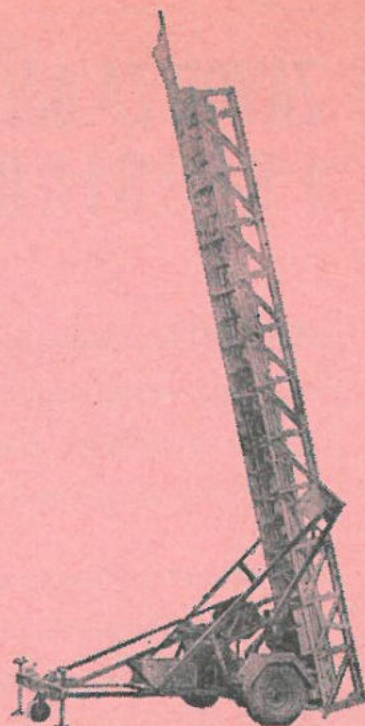
PIL. 18 PRIKOLIČNE IZVLAČNE LJESTVE VERTIKALNE VISINE 10, 12, 15, 18 i 22 m
