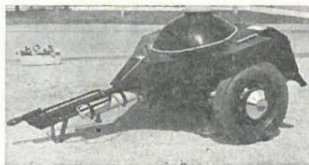
Naš afirmirani aparat (prikolica) tipa S-250, prikladan za brzu vuču i efikasan za gašenje većih požara nastalih paljenjem naftinih derivata
